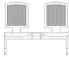
- REKS 322 F Genişlik-Width:100 cm Derinlik-Depth:68 cm Yükseklik-Height:91 cm
